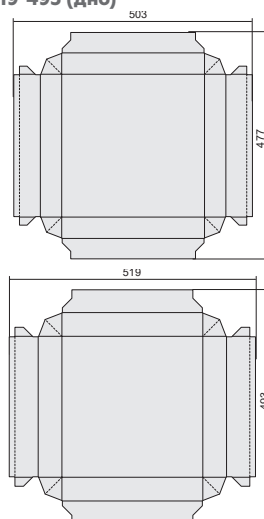
B-169-2A2-3-M1 503*477 (крышка) 519*493 (дно)
