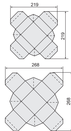
B-26-A4-A3-1-M1 219*219 (крышка) 268*268 (дно)
