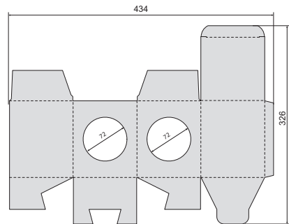
В-133-А3-1с-3-М1 434*326 -упаковка 329*152 -ложемент
