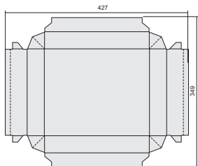
B-150-A3-A2-2c-3-M1 427*349 (крышка) 542*476 (дно)
