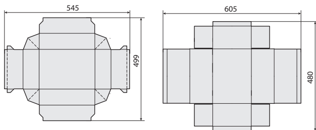
B-29-2A3-D-2-M1 428*268 (крышка) 483*323 (дно)
