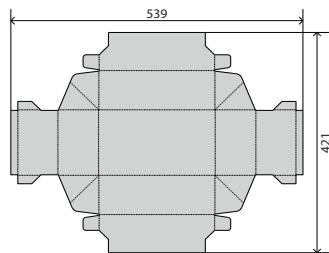
B-134-2A2-3-M1 484*392 (крышка) 499*408 (дно)
