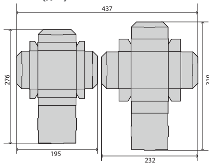
B-241 276*195 (крышка) 310*232 (дно)
