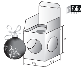
шар d 115мм В-184 126*126*132
