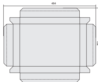
B-134-2A2-3-M1 484*392 (крышка) 499*408 (дно)
