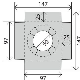
B-99-в-A5-D ложемент в коробку 147*147
